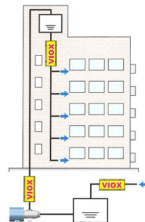
受水槽と高架水槽
